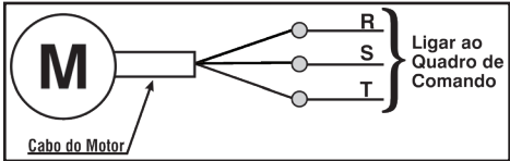
Figura 16a – Esquema de ligação motores trifásicos com 01 cabo chato ou 3 cabos unipolares
