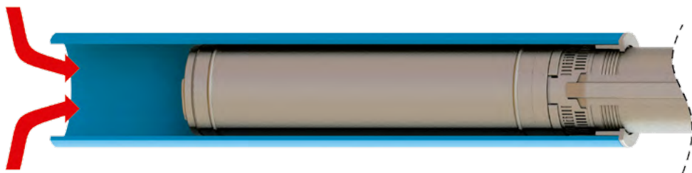
Figura 8: Camisa indutora de fluxo.
