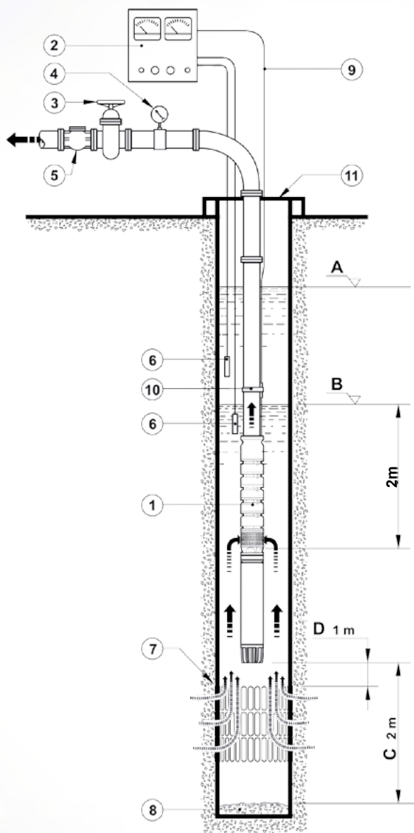
Figura 7: Informações de instalação.
